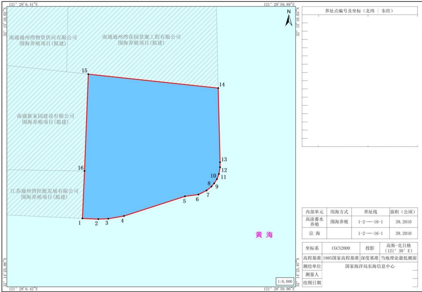
南通清水湾开发有限公司围海养殖用海宗海界址图
