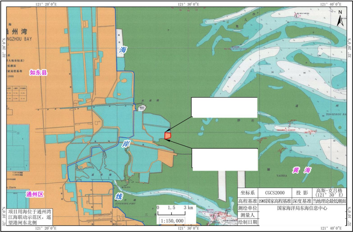
南通清水湾开发有限公司围海养殖用海宗海位置图
