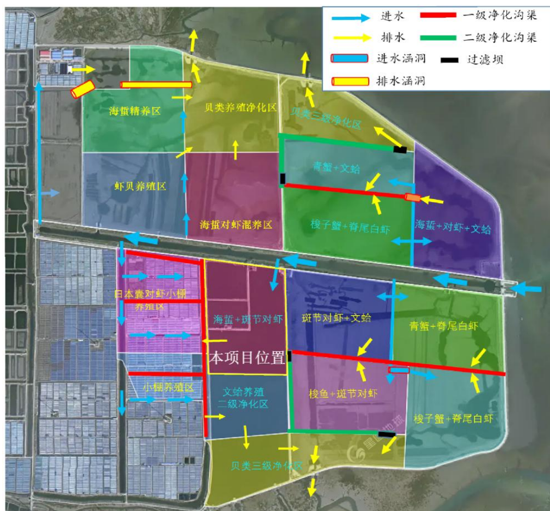
图 1-3 养殖区进排水系设计图
